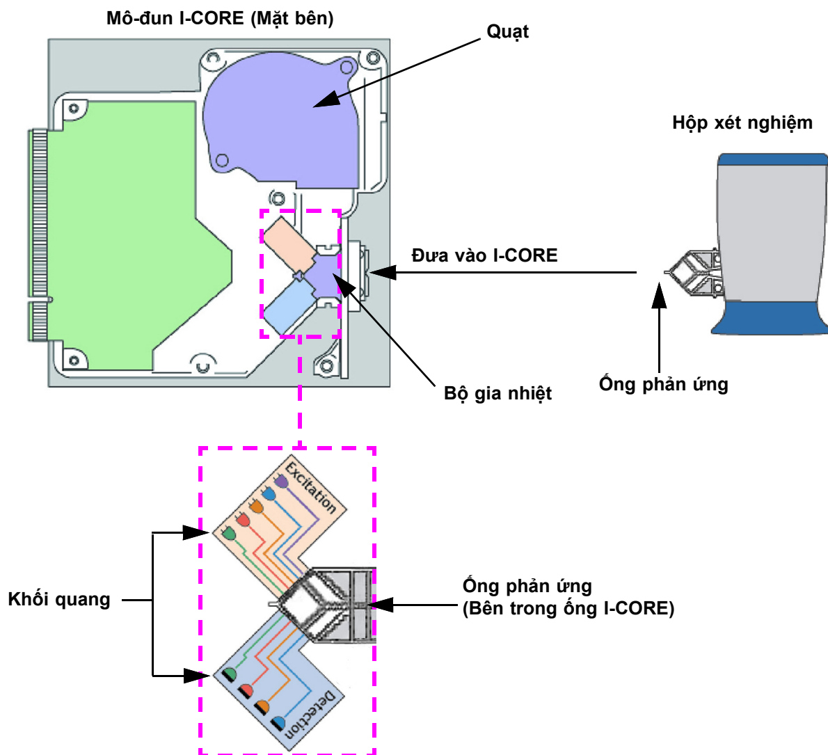
Hình 3-3. Mô-đun I-CORE
