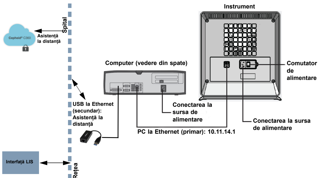
Figura 2-11. Conectarea instrumentului GX-IV la C360
