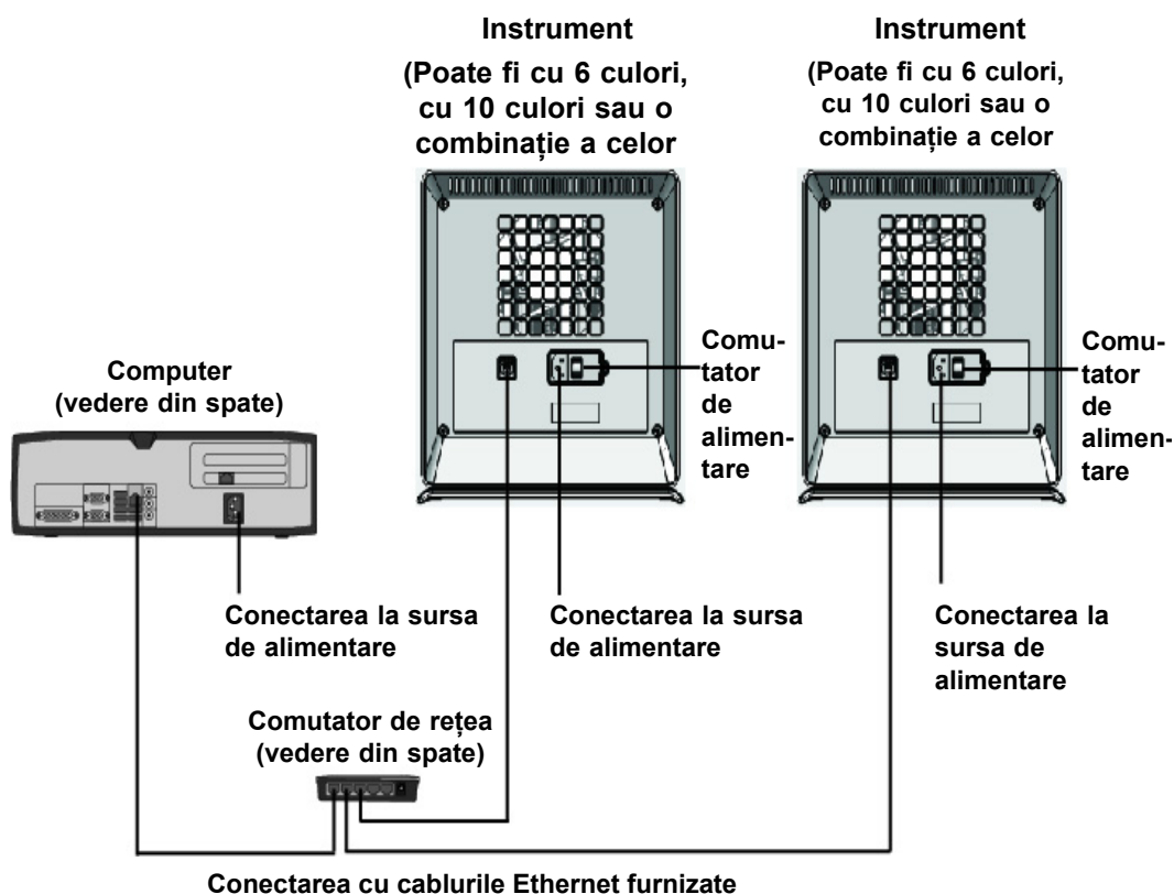
Figura 2-9. Conectarea mai multor instrumente GX-IV la computerul desktop
