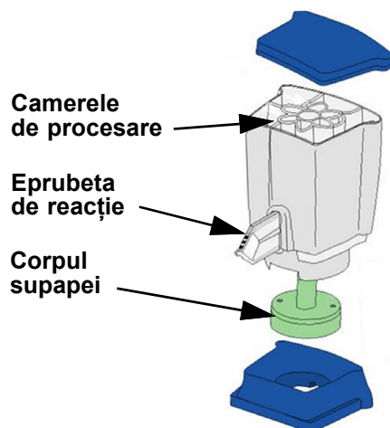
Figura 3-2. Componentele cartușului GeneXpert
