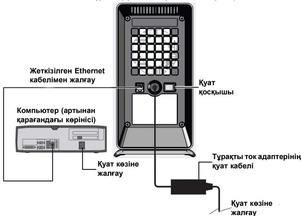
2-2-сурет. GX-II құралын үстел компьютеріне жалғау
