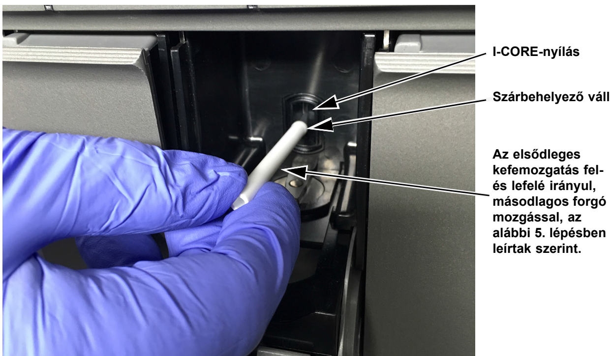
9-7. ábra A tisztítókefe behelyezése az I-CORE nyílásába
