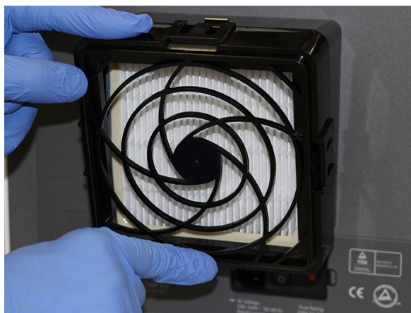
9-30. ábra A HE-szűrő rögzítőelemének cseréje
