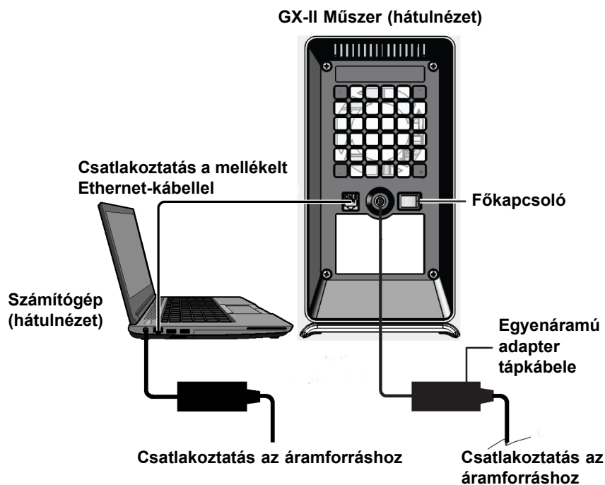
2-6. ábra A GX-II műszer csatlakoztatása a laptop számítógéphez
