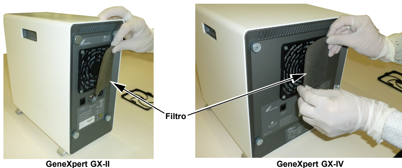
Figura 9-10. Extracción del filtro
