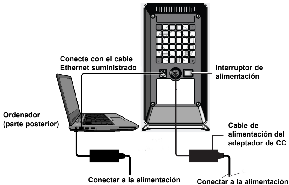
Figura 2-6. Conexión del instrumento GX-II al ordenador portátil
