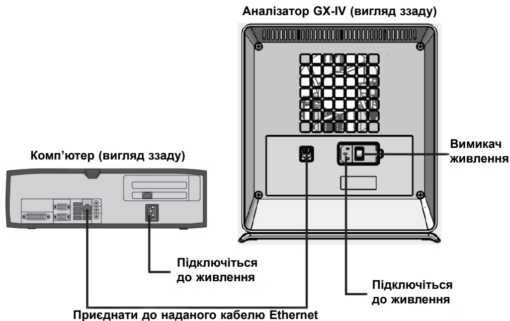
Малюнок 2-3. Підключення аналізатору GX-IV до настільного комп'ютера
