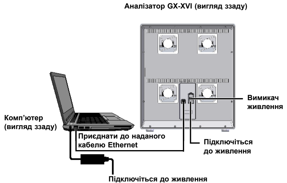
Малюнок 2-8. Підключення аналізатору GX-XVI до переносного комп'ютера
