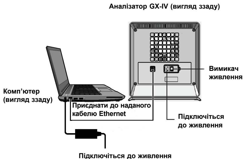
Малюнок 2-7. Підключення аналізатору GX-IV до переносного комп'ютера
