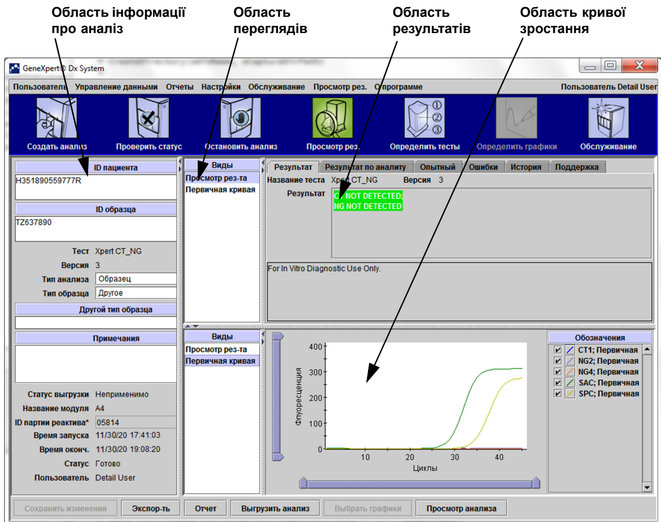
Малюнок 5-41. Вікно GeneXpert Dx Перегляд результатів (Просмотр результатов)—Вкладка Результат анализу (Результат анализа) (Перегляд детальних відомостей про користувачів та адміністратора)
