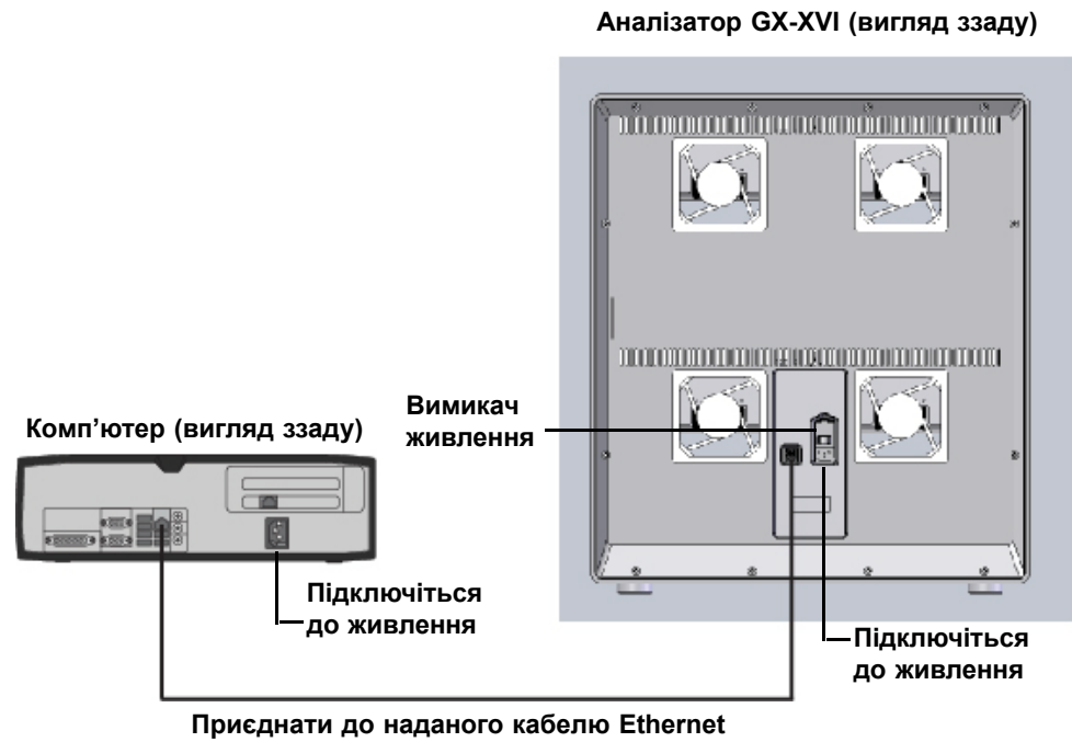
Малюнок 2-4. Підключення аналізатору GX-XVI до настільного комп'ютера
