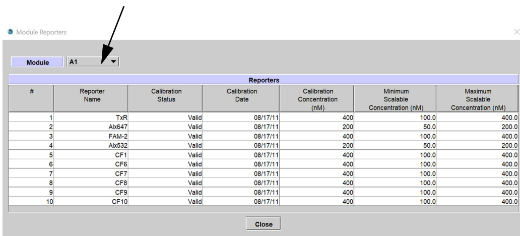
Figur 9-33. Fönster för modulrapporterare som visar en modul med 10-färger
