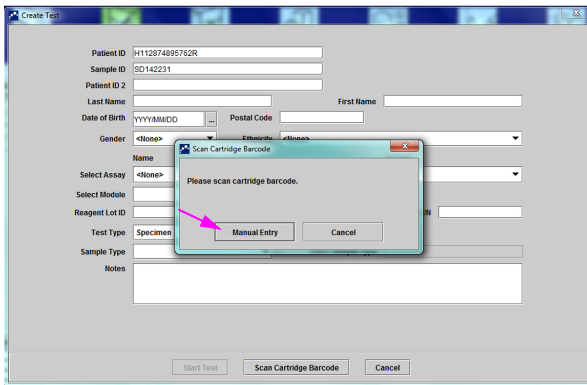
Figur 5-21. Dialogrutan Skanna kassetts streckkod
