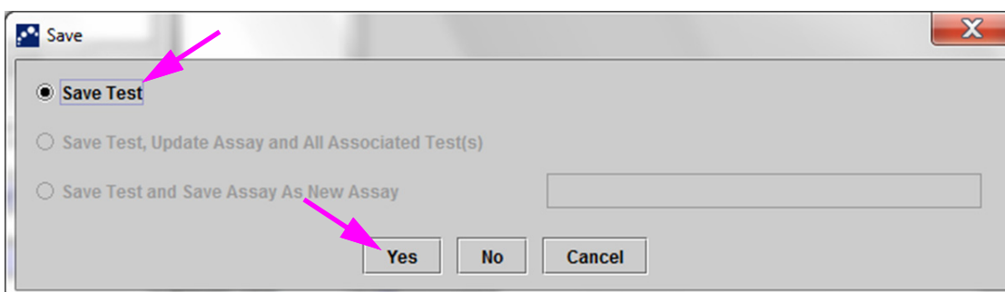
Figur 5-51. Dialogrutan Spara
