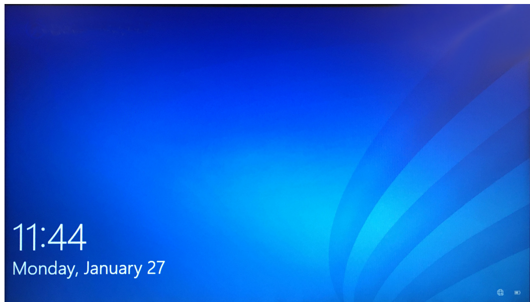
Figur 5-2. Windows 10-låskärmen
