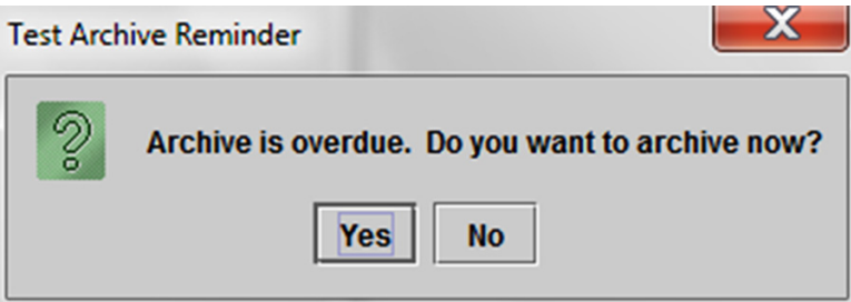
Figur 5-10. Dialogrutan Testarkiveringspåminnelse
