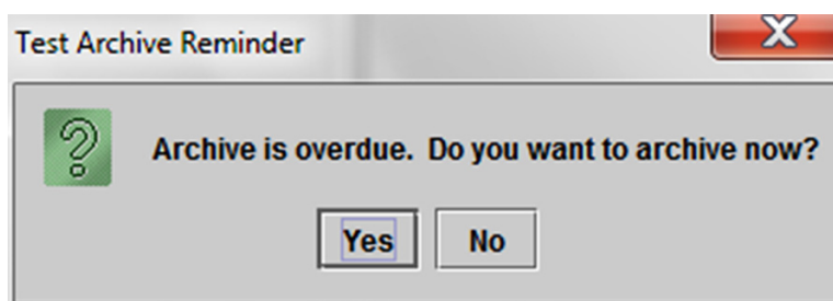
Figur 2-97. Dialogrutan Testarkiveringspåminnelse
