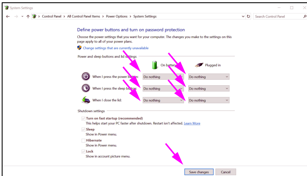
Figur 2-30. Fönstret Systeminställningar
