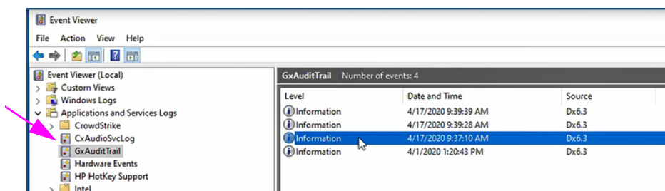
Figur 2-78. Windows händelsegranskare
