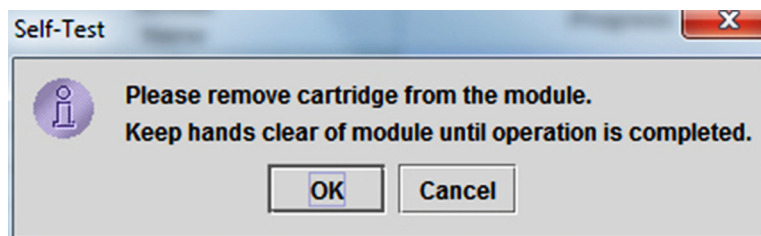
Figur 9-35. Dialogrutan Självtest
