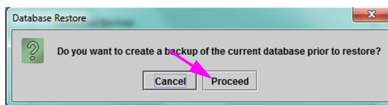
Figur 5-77. Dialogrutan Databasåterställning
