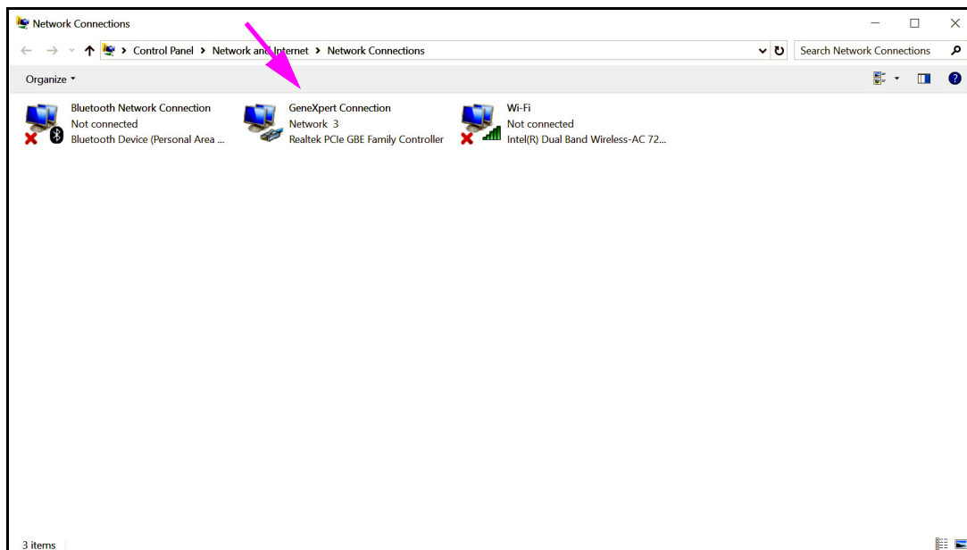
Figur 2-46. Skärmen Nätverksanslutningar
