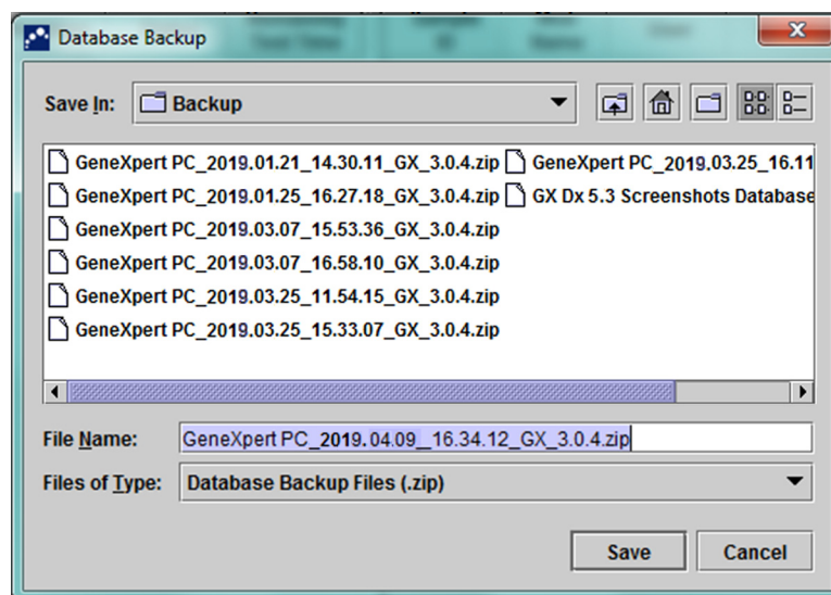
Figur 5-78. Dialogrutan Databassäkerhetskopiering
