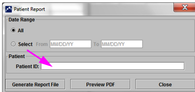
Figur 5-88. Dialogrutan Patientrapport
