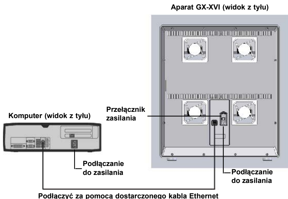
Ilustracja 2-4. Podłączanie aparatu GX-XVI do komputera stacjonarnego
