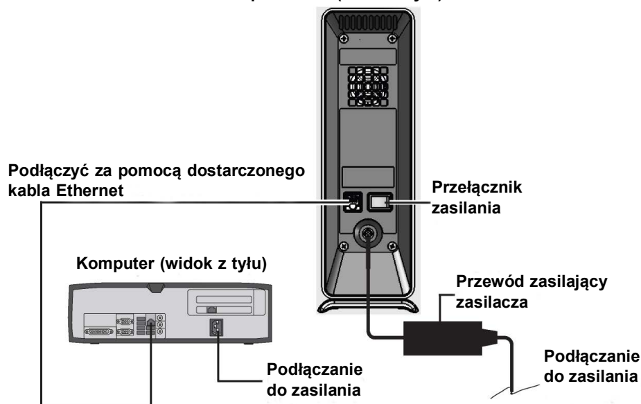
Ilustracja 2-1. Podłączanie aparatu GX-I do komputera stacjonarnego
