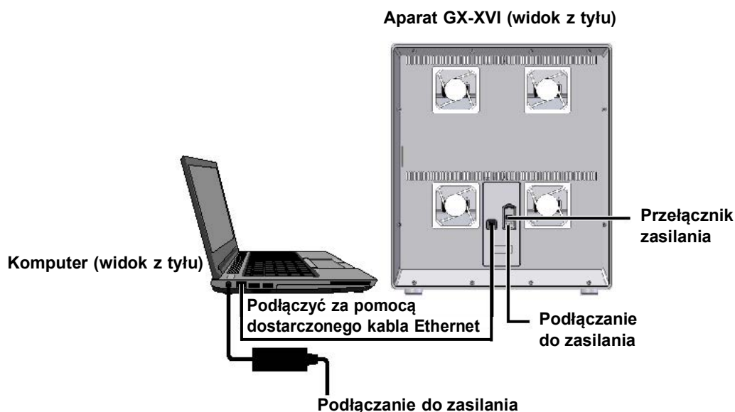
Ilustracja 2-8. Podłączanie aparatu GX-XVI do laptopa
