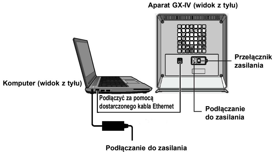
Ilustracja 2-7. Podłączanie aparatu GX-IV do laptopa
