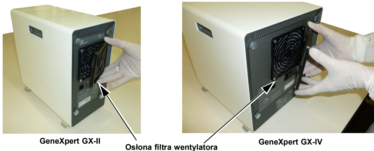
Ilustracja 9-9. Zdejmowanie osłony filtra wentylatora
