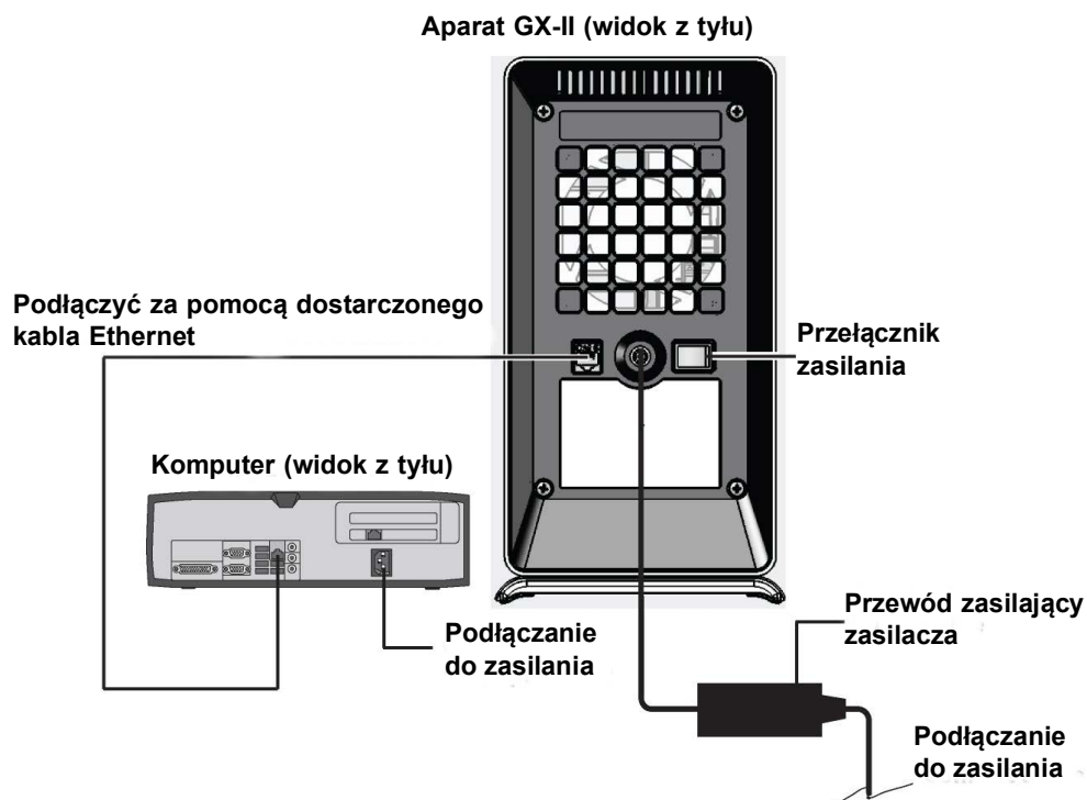
Ilustracja 2-2. Podłączanie aparatu GX-II do komputera stacjonarnego
