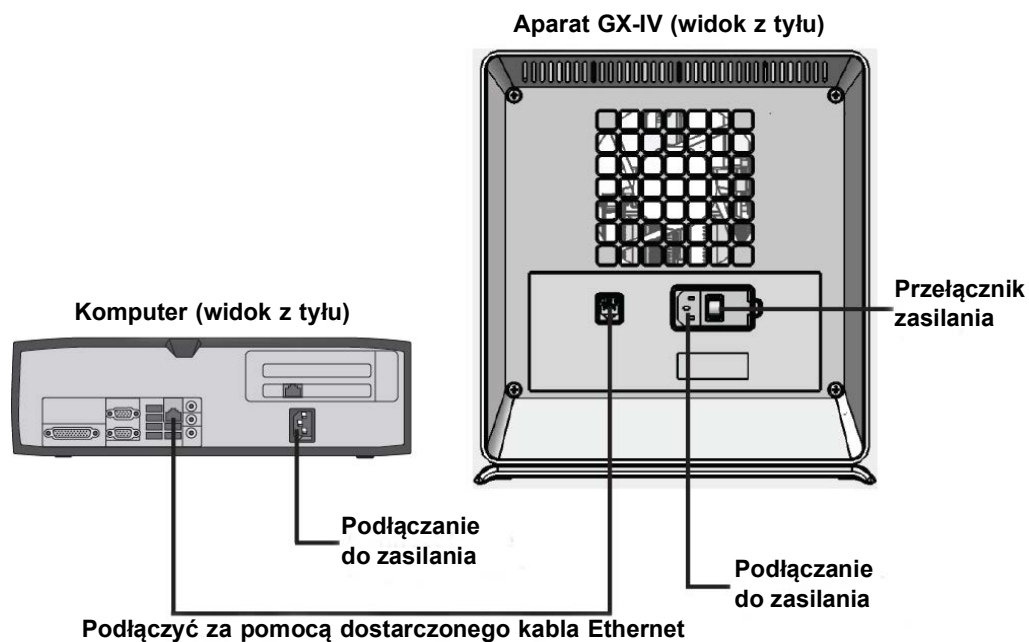
Ilustracja 2-3. Podłączanie aparatu GX-IV do komputera stacjonarnego
