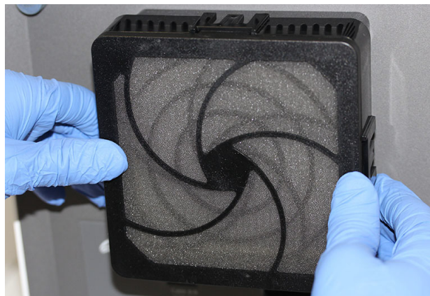
9-31. attēls. Priekšfiltra un priekšfiltra aiztura nomaiņa
