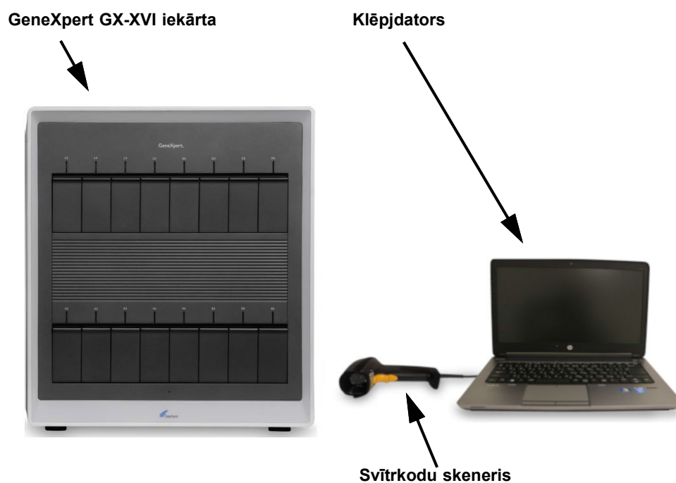
1-8. attēls. GeneXpert GX-XVI aparātūras komponenti (parādīti ar klāpjdatoru)
