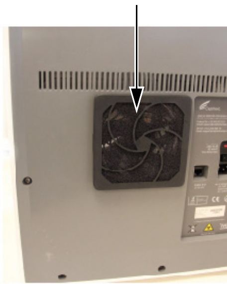
9-23. attēls. Filtra un aizsarga nomaiņa
