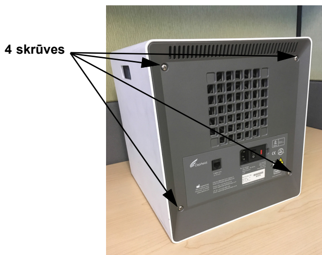
9-14. attēls. Aiz mugures paneļa skrūves vecākā GX-IV modelī
