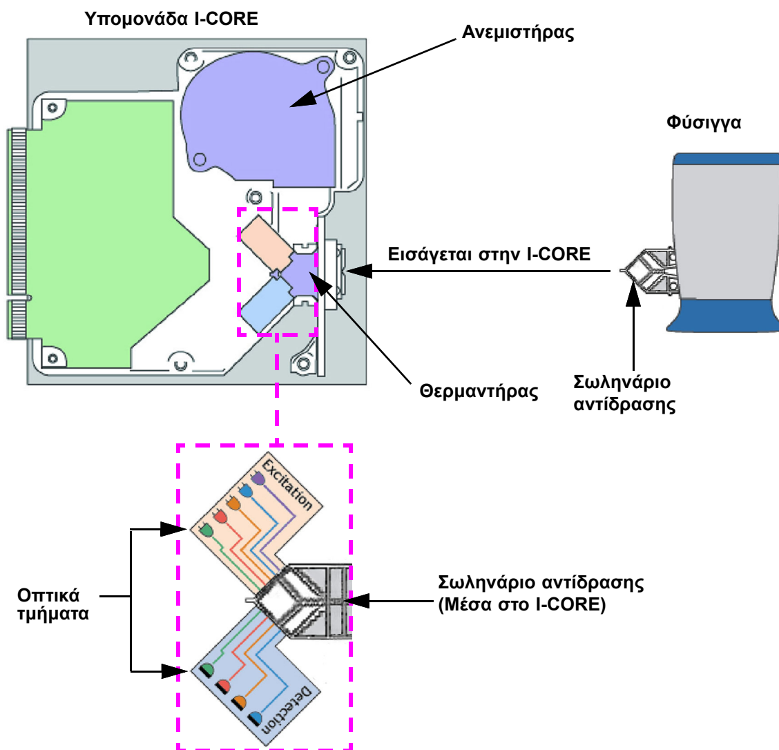
Εικόνα 3-3. Υπομονάδα I-CORE
