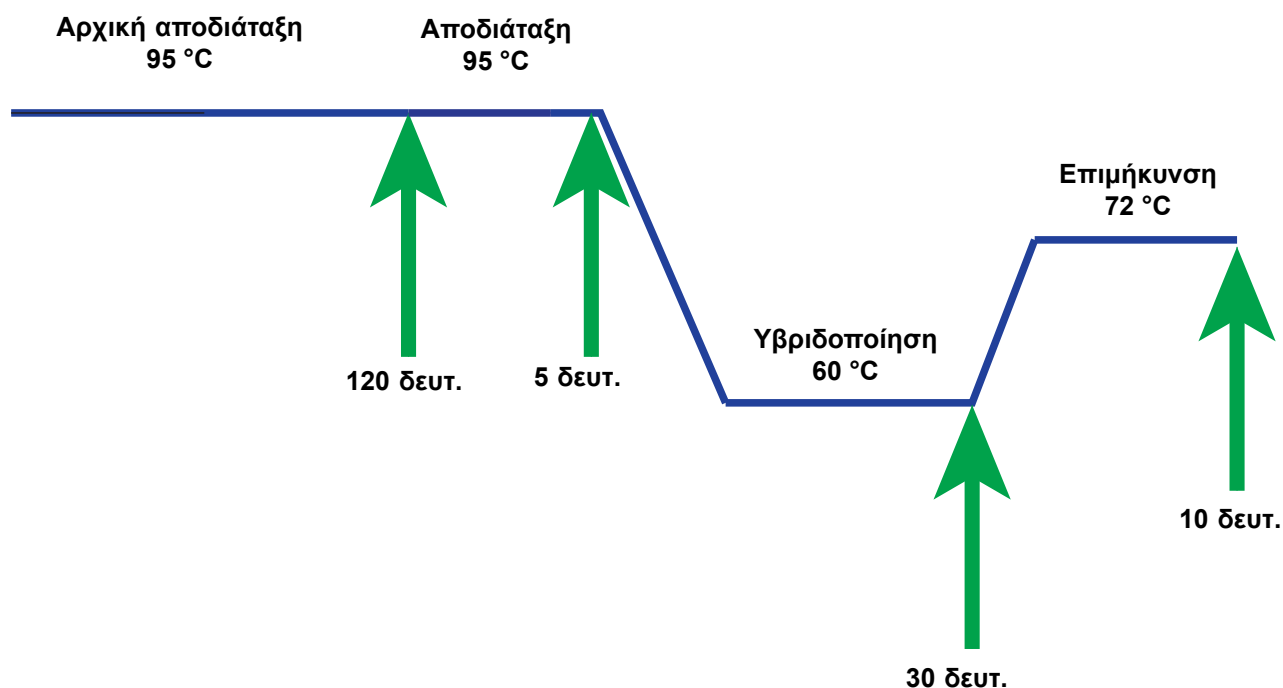
Εικόνα 3-1. Διάγραμμα παραδείγματος κύκλου PCR για τη θέρμανση και την ψύξη με ανεμιστήρα της υπομονάδας I-CORE (Οι διάρκειες των θερμοκρασιών δεν είναι σε κλίμακα)
