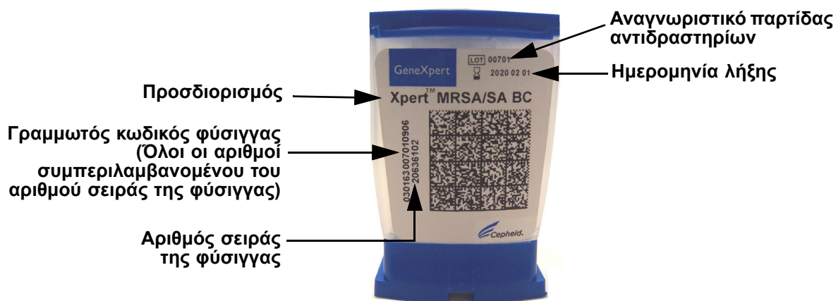
Εικόνα 5-22. Φύσιγγα GeneXpert
