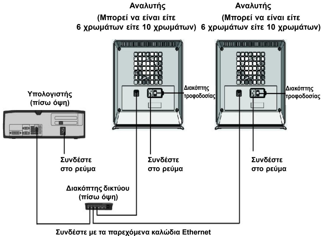
Εικόνα 2-9. Σύνδεση πολλαπλών αναλυτών GX-IV σε σταθερό υπολογιστή
